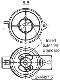
KLEMMSOCKEL
