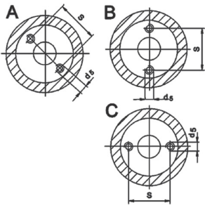
KLEMMSOCKEL
